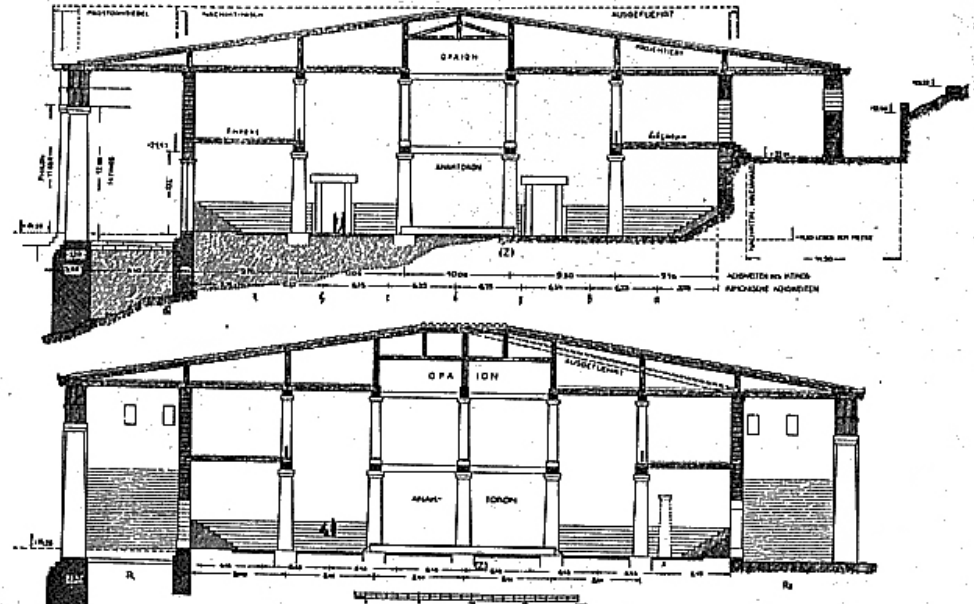
Fig. 76. Telesterion, Eleusis; proyecto de Ictino, conjeturalmente reconstruido. (a) arriba: sección este-oeste, con indicación adicional del proyecto en realidad terminado, incluyendo el pórtico de Filón. (b) abajo: sección norte-sur, con indicación adicional de la mitad de la derecha (norte) del proyecto de cubierta que se llegó a realizar, así como de una de las columnas interiores posteriores (x). Bajo cada figura se ofrece una comparación entre los intercolumnios del proyecto de Ictino y el anterior, de Cimón, con las medidas interaxiales
